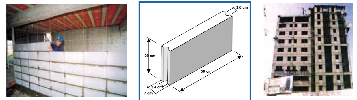
Fig. 1. Uso de la Placa P-7 en la construcción de tabiques permanentes (fijos).
