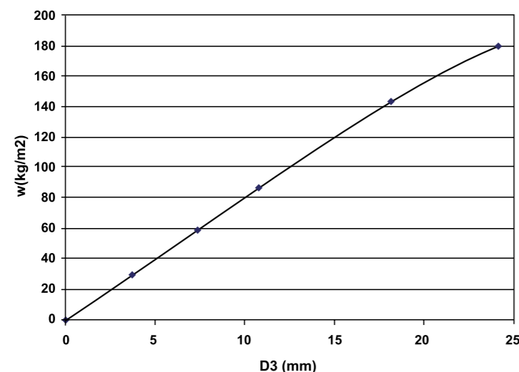
Fig.9 Curva w-D3 en las 5 fases del ensayo sísmico.
