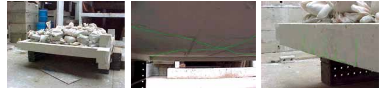
Fig.10. Ensayo estático (izq.), fisuras en el tabique (centro) y fisuras en la columna (der.).
