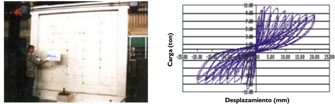
Fig.6. Estado final del conjunto y gráfica cortante-desplazamiento lateral.
