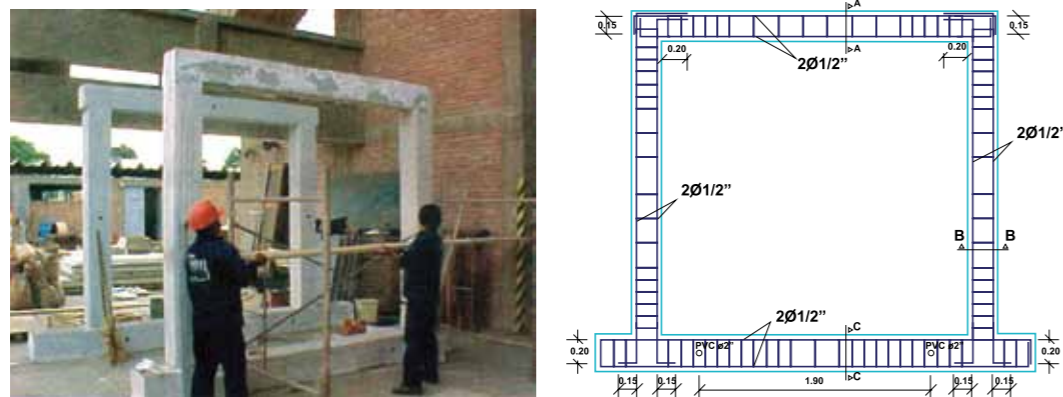
Fig.2 Pórticos de concreto armado.
