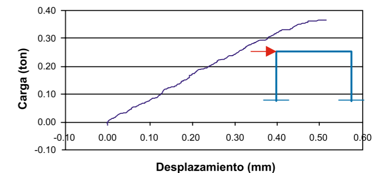
Fig.5 Ensayo monotónico del pórtico en el rango elástico.
