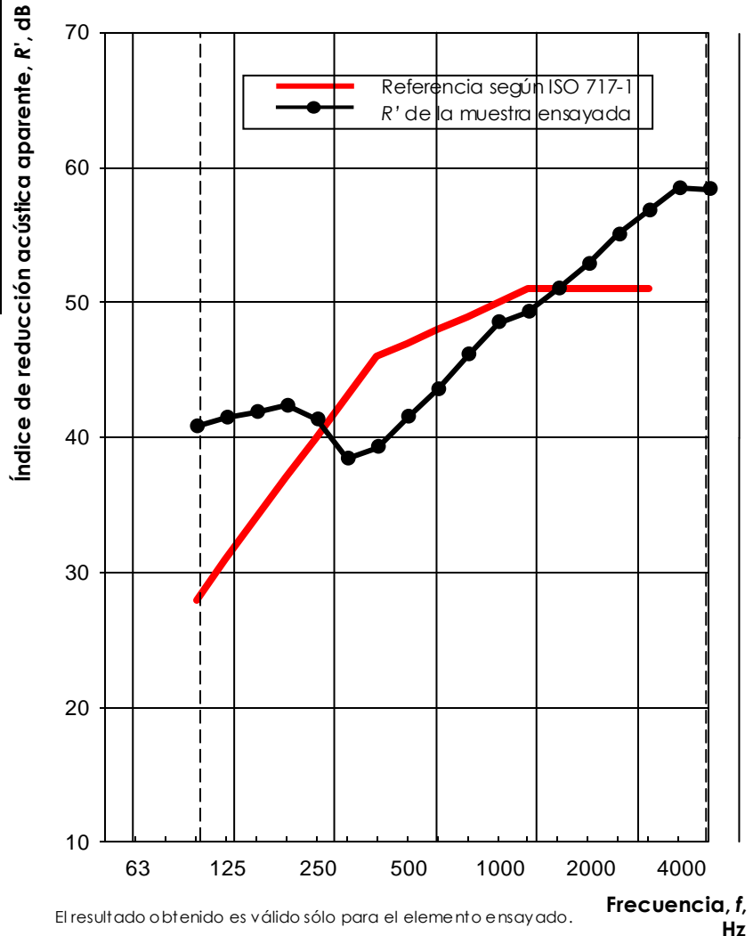
Placa P-12
